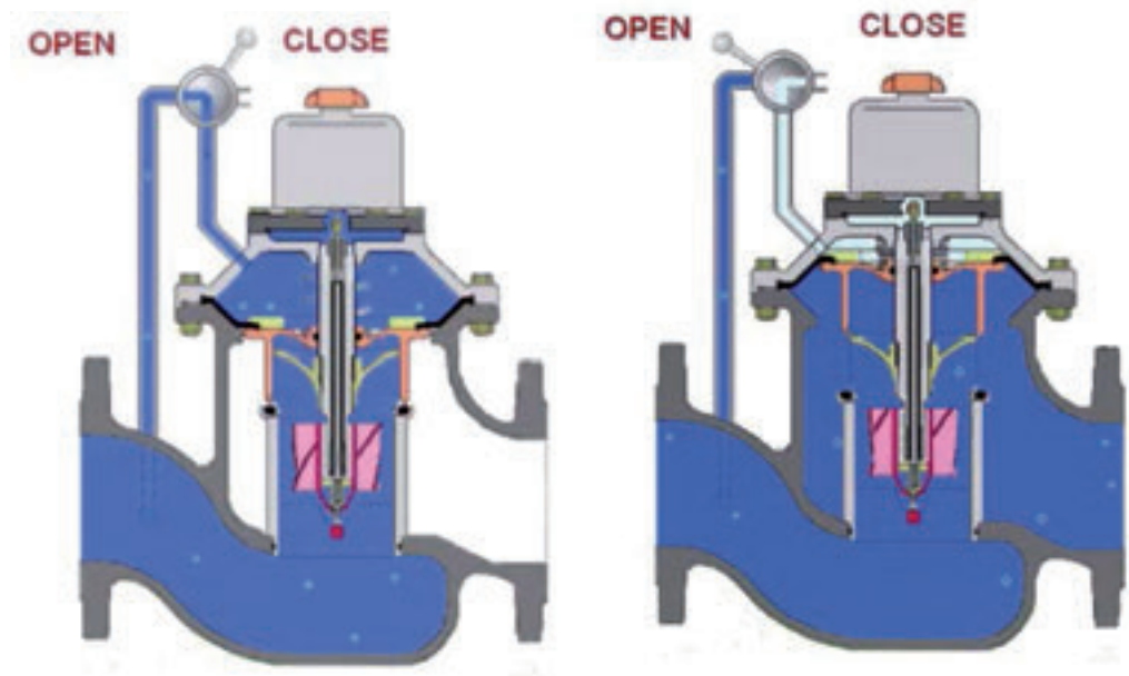
Imagen 13: válvula contador seccionada cerrada y abierta. Fuente Bermad.
