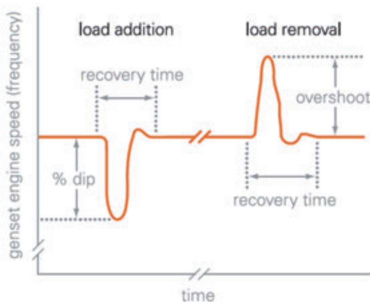
Figura 6. Transitorio arranque-paro.
