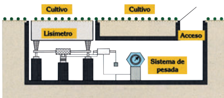
Figura n.º 1: Esquema de un lisímetro de pesada.
