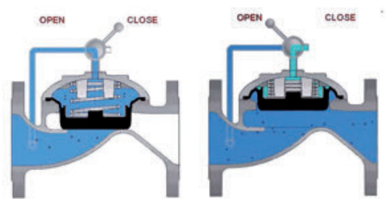
Imagen 2: Válvula hidráulica seccionada cerrada y abierta. Fuente Bermad.
