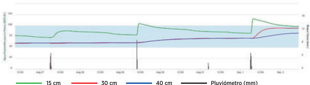
FIGURA 4. Gráfica de seguimiento de la evolución del suelo del día 2 de septiembre enviada al agricultor de uno de los demostradores. En la gráfica se muestra la aportación de 3 riegos que elevan la humedad a 15 cm de profundidad sin apenas elevar la humedad del suelo a 40 cm, de forma que en esta semana no se produjeron pérdidas por percolación.
