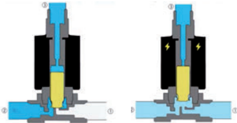
Imagen 6: Solenoide de imán-bobina en posición de reposo y accionado. Fuente Baccara.
