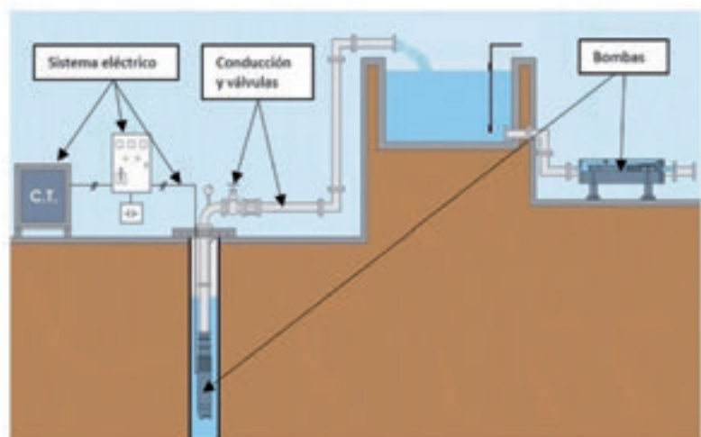
Elementos significativos de un bombeo.
