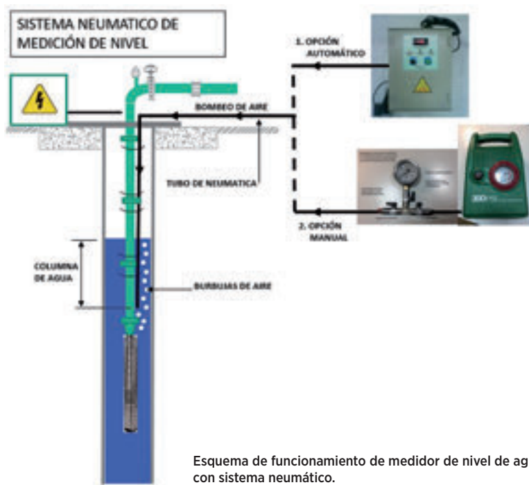
Medidor de nivel neumático. Distribuidor: JUAN AZCUE S.A.
