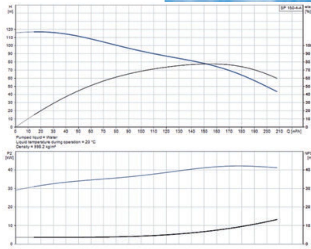
Curvas de una electrobomba sumergida.
