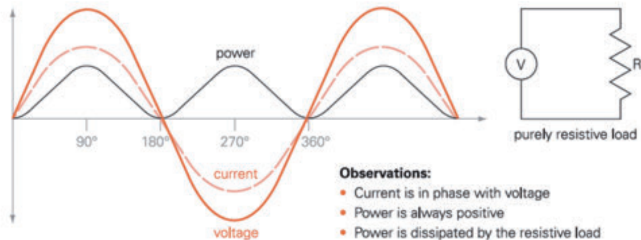
Figura 3. Carga resistiva.
