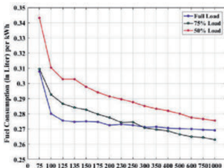
Figura 2. Consumo específico según tamaño generador a diferentes cargas.
