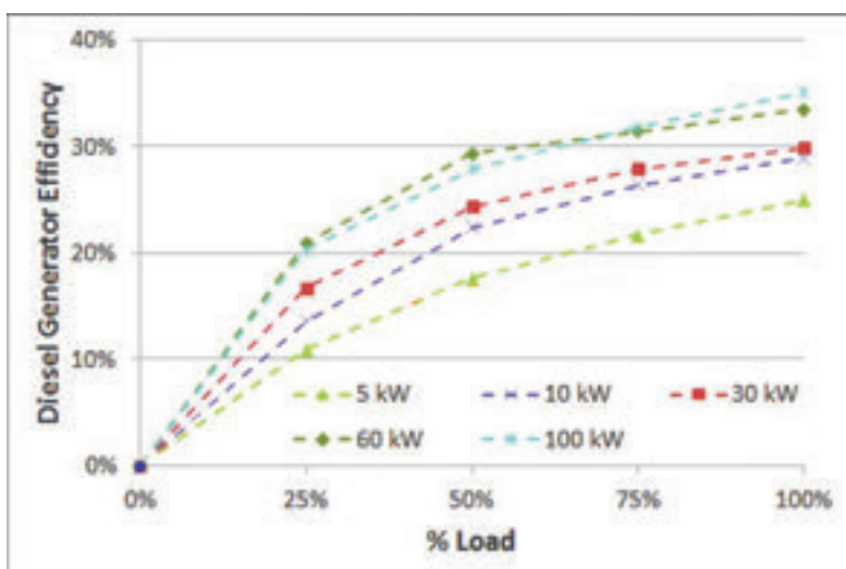
Figura 1. Eficiencia según carga para diferentes potencias.
