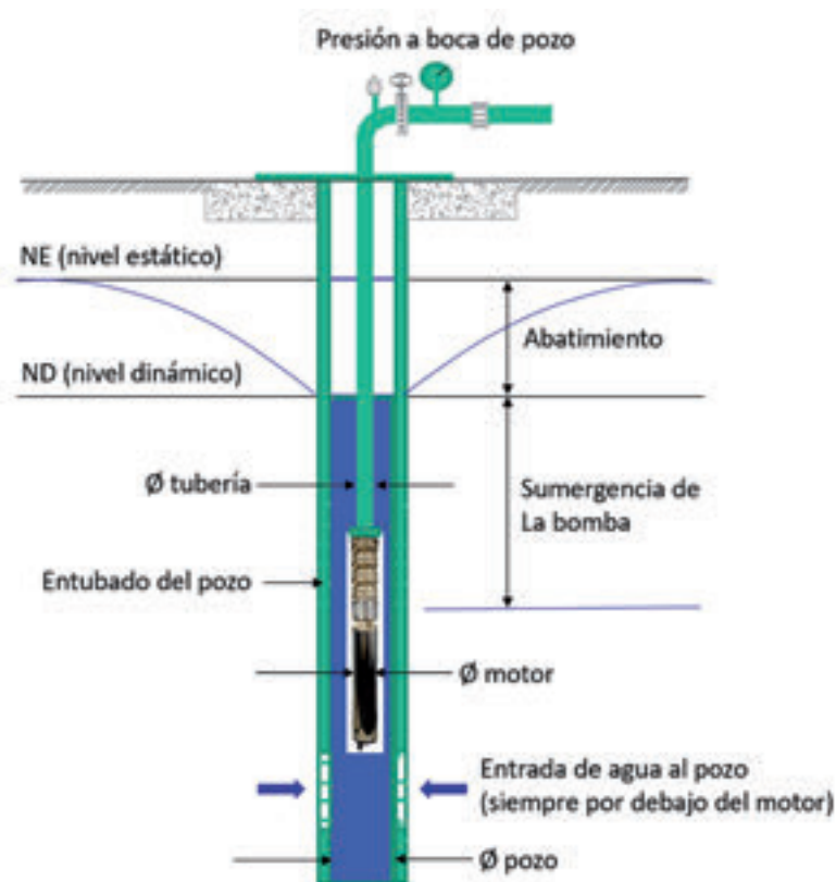
Croquis de un pozo.
