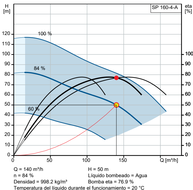
Curvas de consumo de una bomba a diferentes frecuencias de trabajo.
