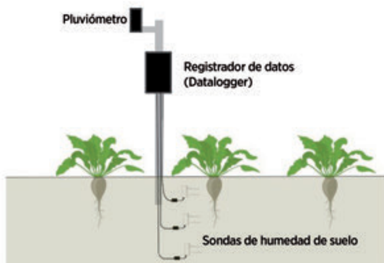
FIGURA 2. Esquema de un punto de control de humedad del suelo, formado por 3 sondas de humedad de suelo, un registrador de datos que envía la información vía GPRS y un pluviómetro para detectar los aportes de agua (riego o lluvia). Los dos sensores más superficiales aportan información de la zona de mayor actividad radicular. El tercer sensor, colocado a mayor profundidad, mide el contenido de humedad fuera de la zona de mayor influencia de las raíces.
