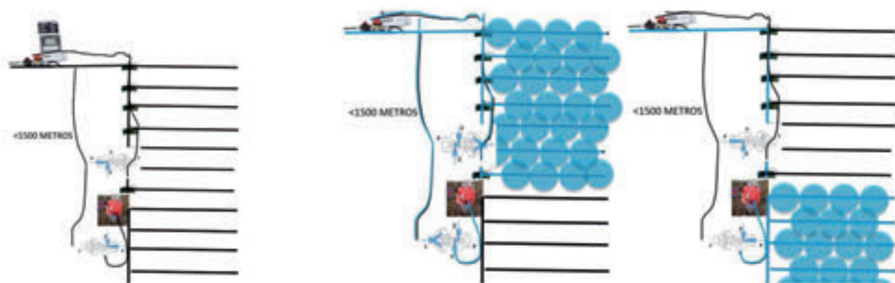
Imagen 16: secuencia de manejo de dos sectores con un programador de una salida y un refuerzo de señal dentro del sector. Fuente elaboración propia.
