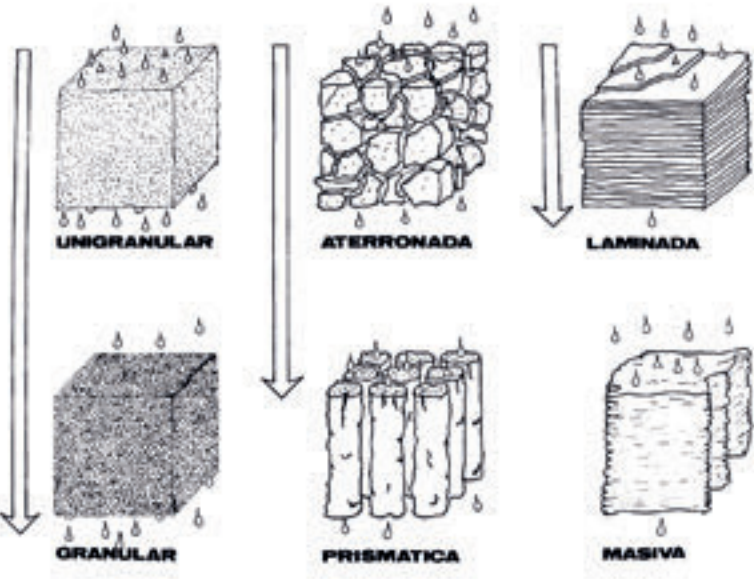
La estructura del suelo condiciona su permeabilidad.
