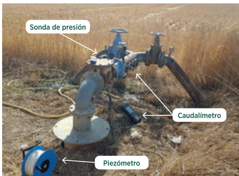
Medida parámetros hidráulicos (caudal, presión y nivel de agua dinámico) con equipos portátiles no invasivos.
